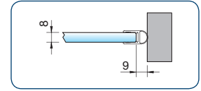
Art.-Nr. 8861KU7-8-2010 Dichtprofil für den seitlichen Wand- anschluss 90° (Beschlagseite) für 6 und 8 mm Glas für ein- und beidseitig zu öffnendes Duschtürband
