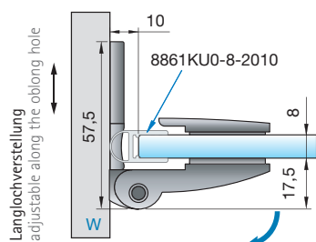
8128ZN mit Dichtprofil 8861KU0-8-2010 8128ZN with sealing profile 8861KU0-8-2010
