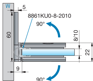
8406MS mit Dichtprofil 8861KU0-8-2010 8406MS with sealing profile 8861KU0-8-2010
