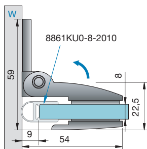
8120ZN mit Dichtprofil 8861KU0-8-2010 8120ZN with sealing profile 8861KU0-8-2010
