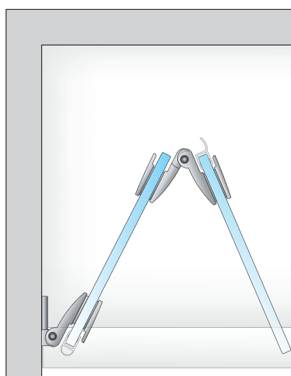
maximale Ausladung bei einer Höhe von 1600mm beträgt 1400mm Having a height of 1600mm the maximum width is 1400mm
