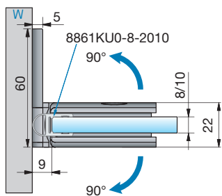
8406MS mit Dichtprofil 8861KU0-8-2010 8406MS with sealing profile 8861KU0-8-2010
