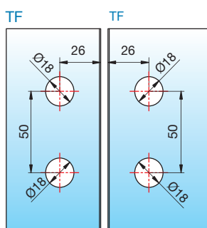
Glasbohrung glass bore
