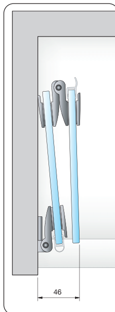
8122ZN mit Dichtprofil 8857KU0-8-2010 8122ZN with sealing profile 8857KU0-8-2010
